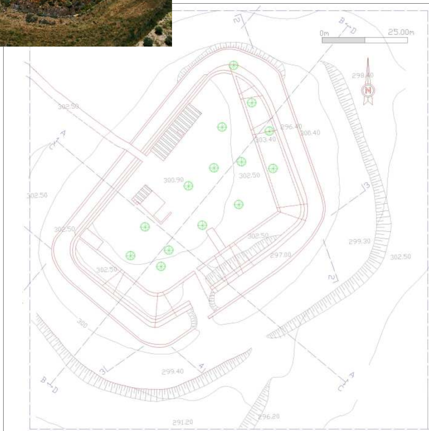
Fig. 1.e 7 – Planta do Fortim de São Mamede Fortlet of São Mamede plan
