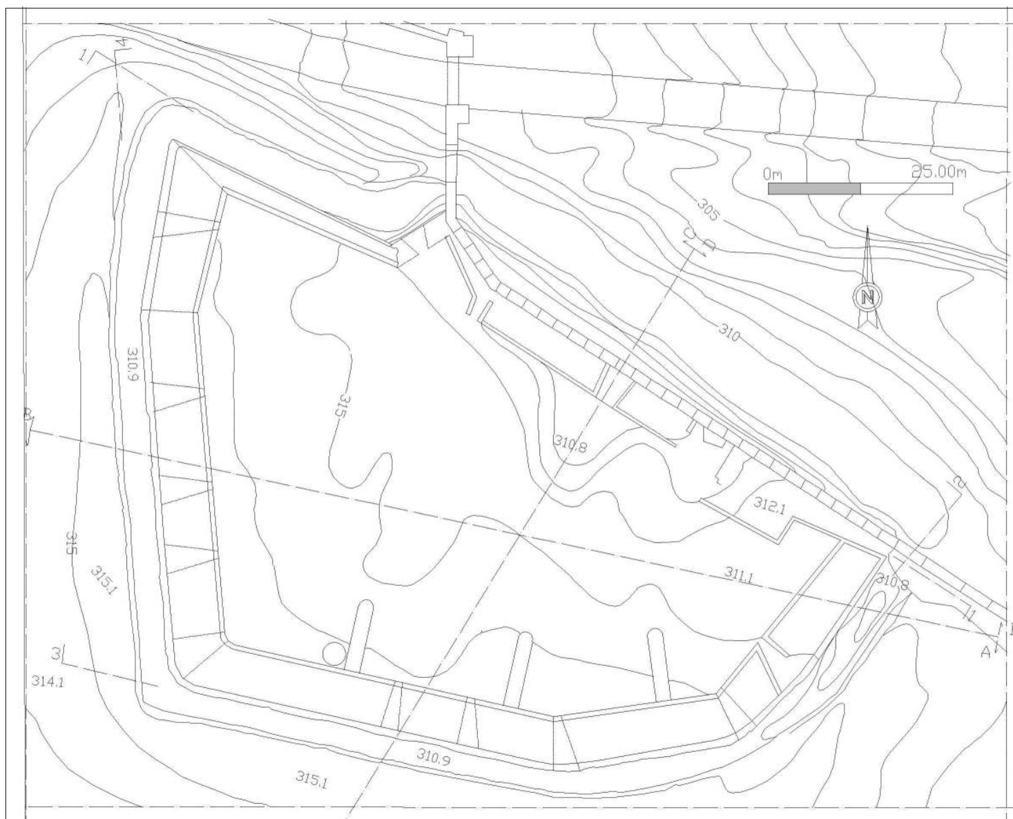
Fig. 1.e.9 – Planta do Fortim de São Domingos ou da Piedade Fortlet of São Domingos or of Piedade plan
